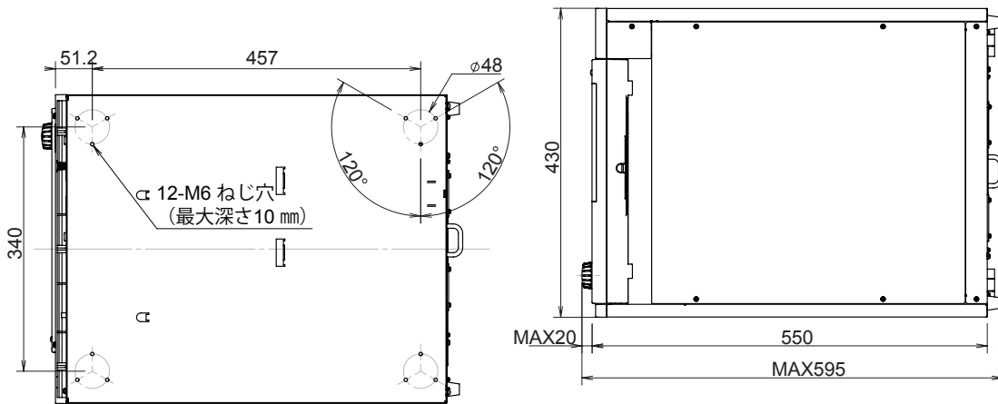
A矢視キャスタねじ位置図
